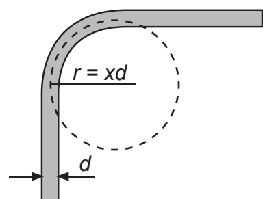
Изгиб провода ПуВ и АПВ
